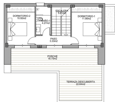
PLANTA PRIMERA
