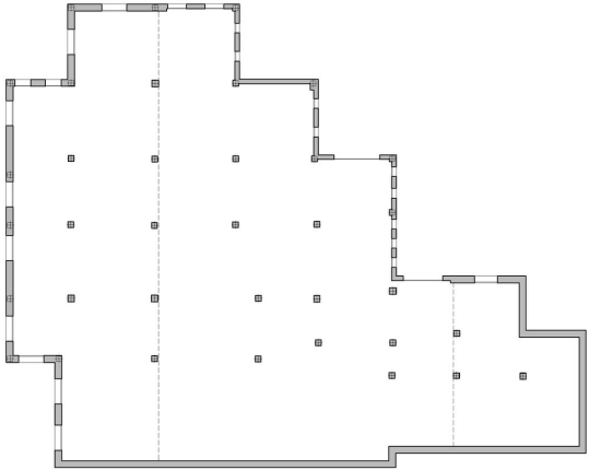
Planta cota -5.40
