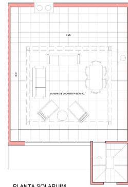
PLANTA SOLARUIM
