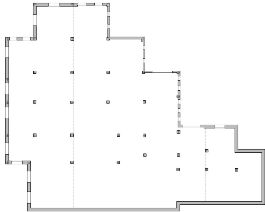
Pianta cota -5.40
