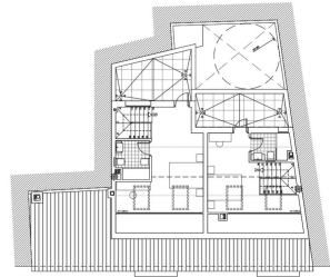
PLANTA BAO CUBERTA
