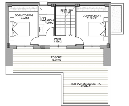
PLANTA PRIMERA
