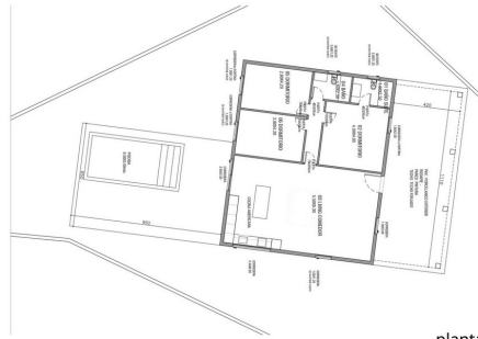
planta propuesta
