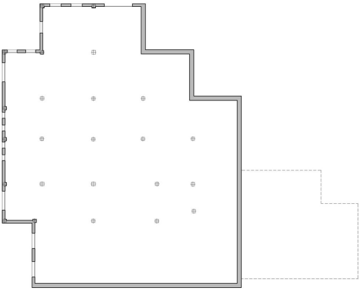
Pianta cofa -9.48
