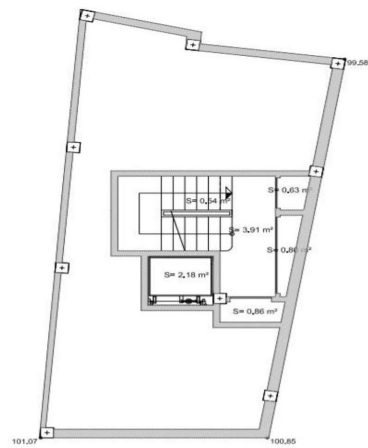
Plano Entrepanta
